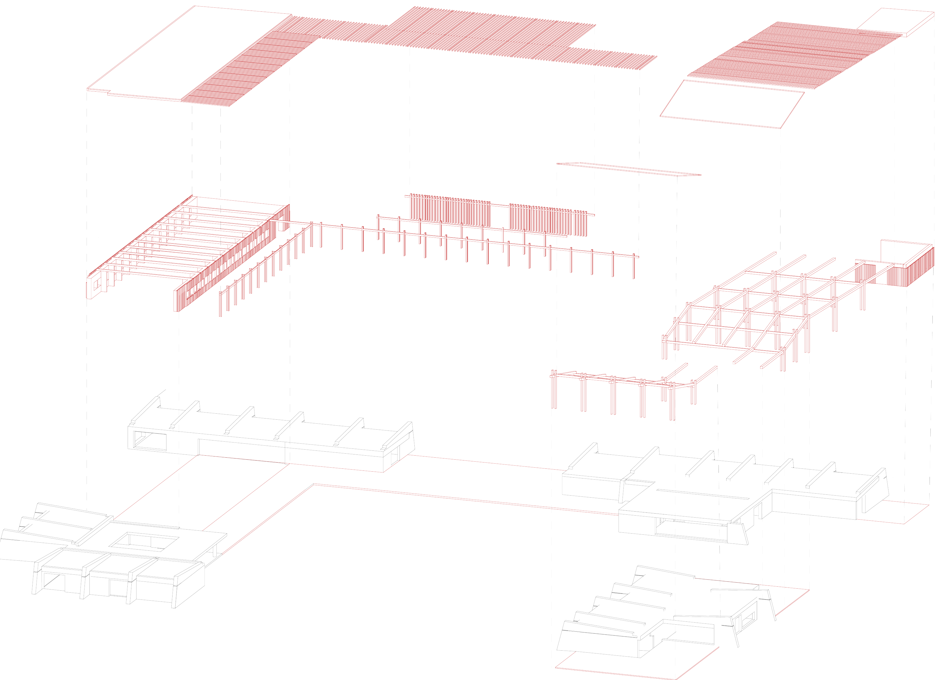
AXONOMÉTRIE STRUCTURELLE
